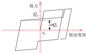
图 7 剪切本构 Fig.7 Horizontal shear spring model
