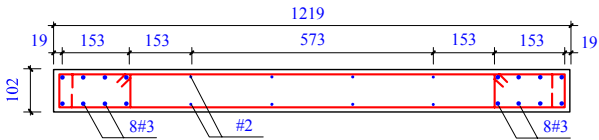
图 13 试件 RW2 配筋图 Fig.13 Details of specimen Spec.RW2
