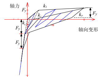
图5 Kabeyasawa 弹簧本构
