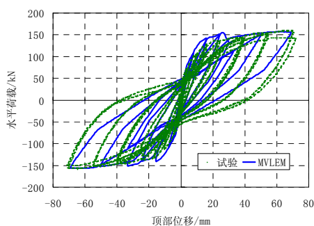
(b) 基于 Fischninger 弹簧本构
