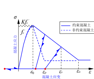
图3 Kent-Park 混凝土本构
