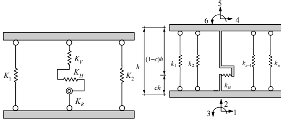
图1 TVLEM 模型示意图 图2 MVLEM 模型示意图 Fig.1 Sketch of TVLEM Fig.2 Sketch of MVLEM
