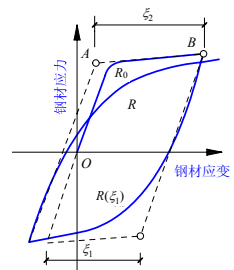
图4 Pinto 钢筋本构
